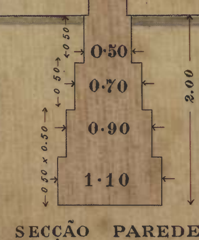
SECÇÃO PAREDE
