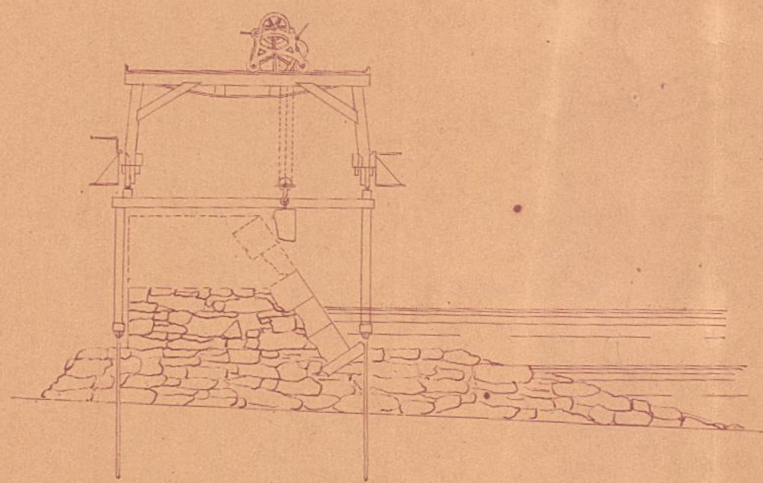
SEÇÃO AB.
