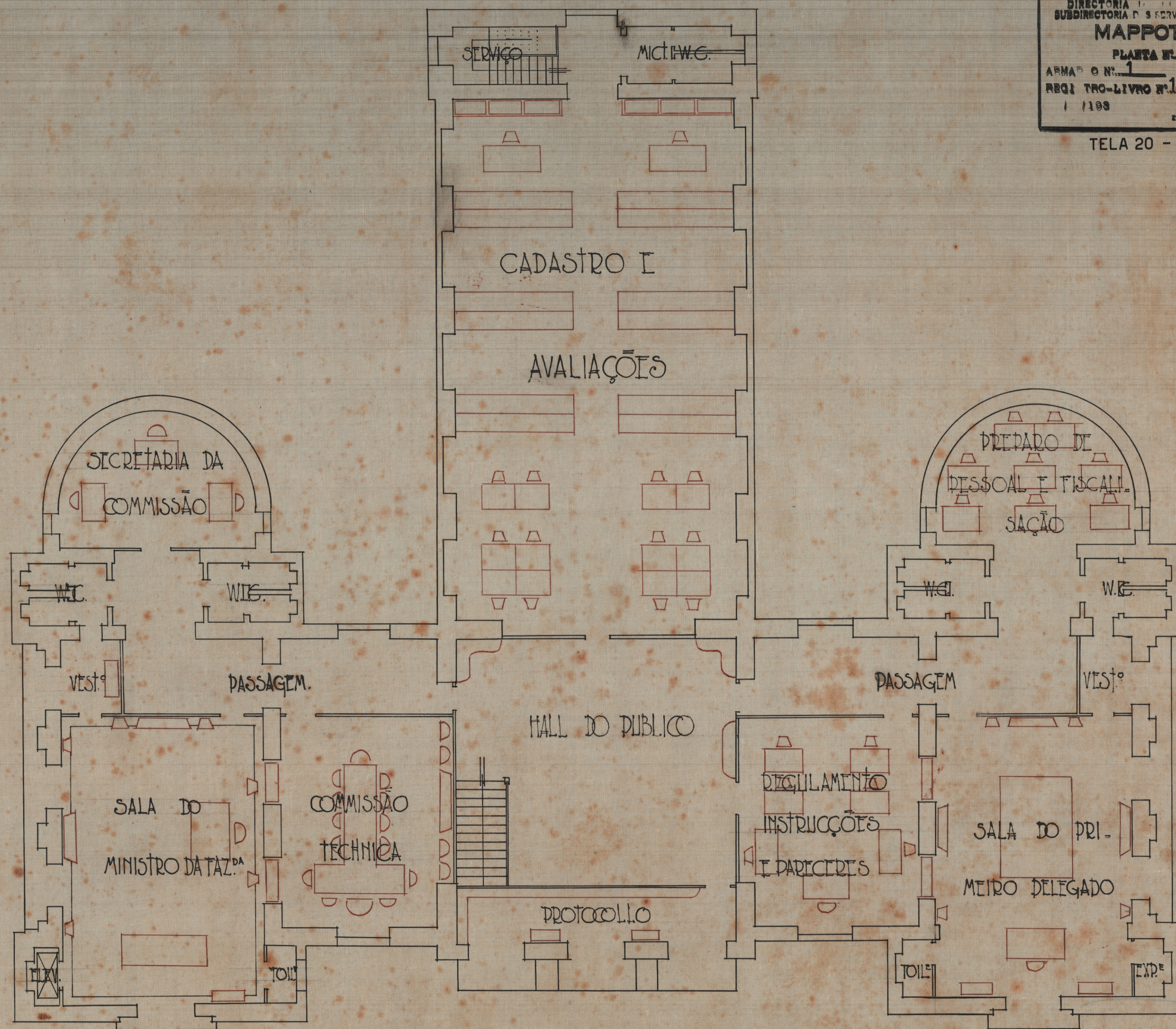
PLANTA DO 2.º PAVIMENTO
